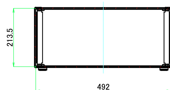
A-A ( 1 : 8.5 )
