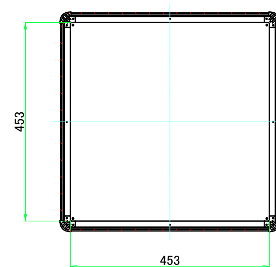
C-C ( 1 : 8.5 )
